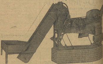
Debulhador de milho com alimentador automático
