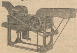
Debulhador com alimentador manual
